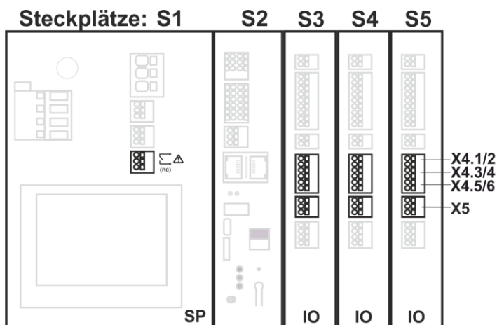
Beispiel: RWA-Zentrale mit 3 x Input/Output-Modulen
