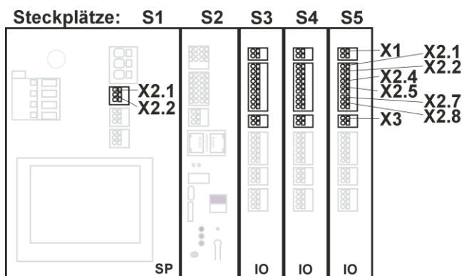
a) RWA-Zentrale mit drei Input/Output-Modulen
