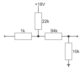
Eingangsschaltung (vereinfacht)
