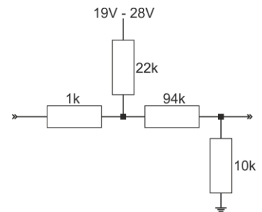
Circuit d'entrée (simplifié)
