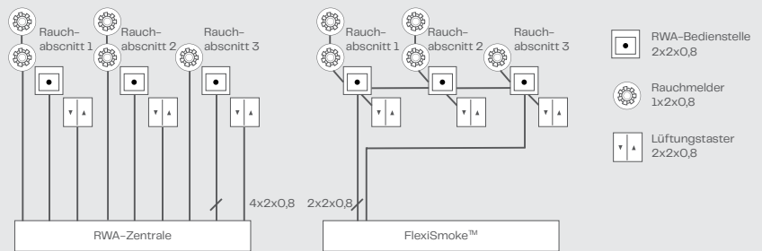
Typische Verkabelungsführung
