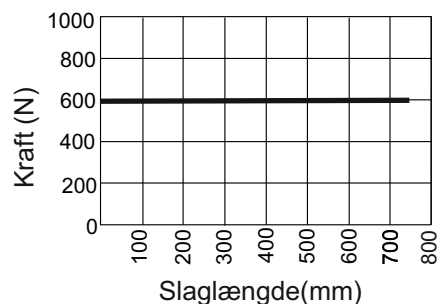
Kraft-slaglængde diagram
