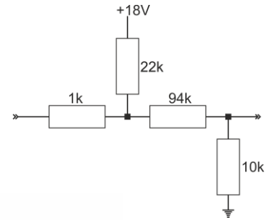
Eingangsschaltung (vereinfacht)
