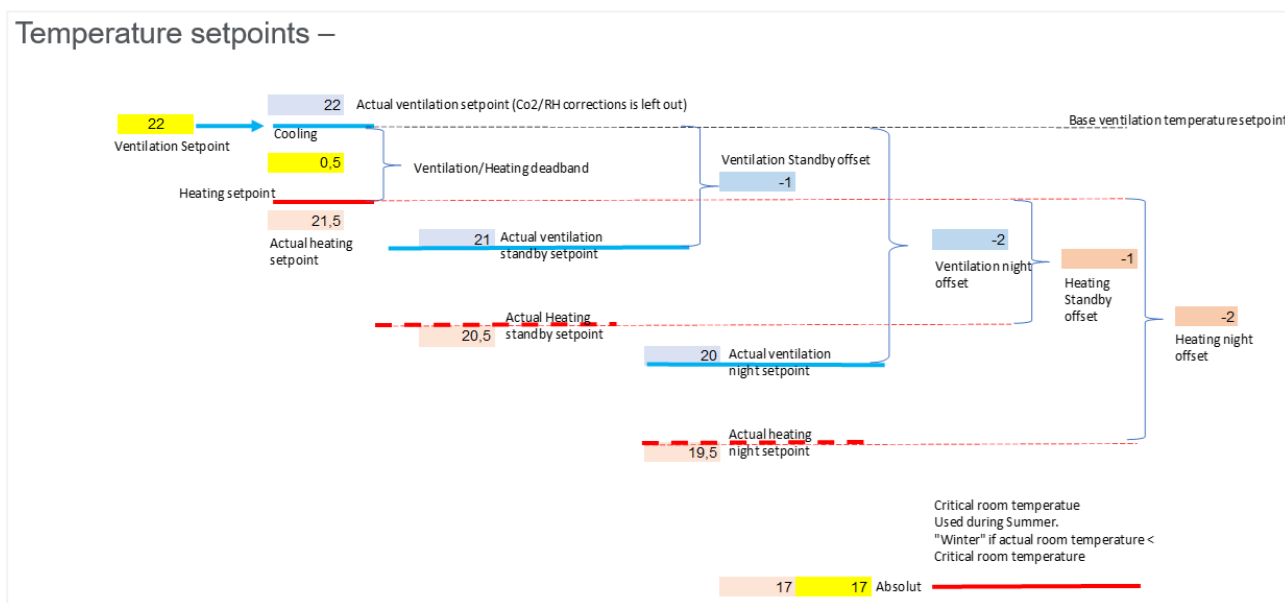
Temperatursætpunktsmodel
