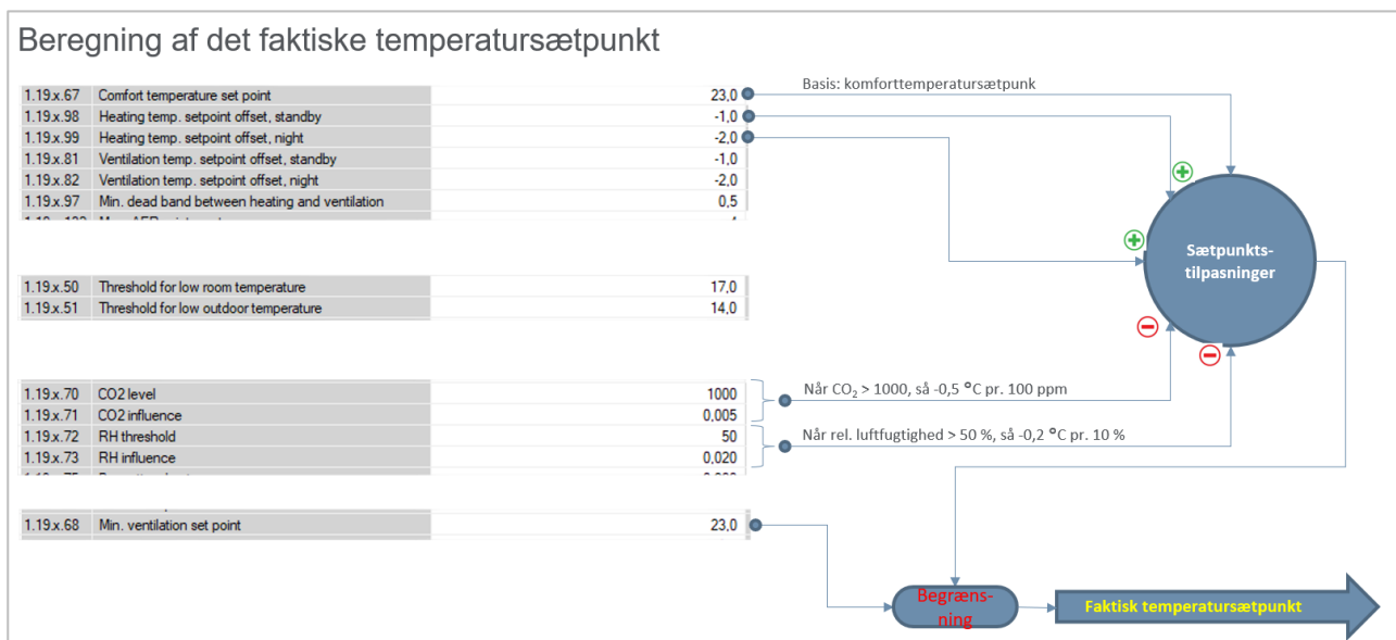
Faktisk temperatursætpunktsberegning
