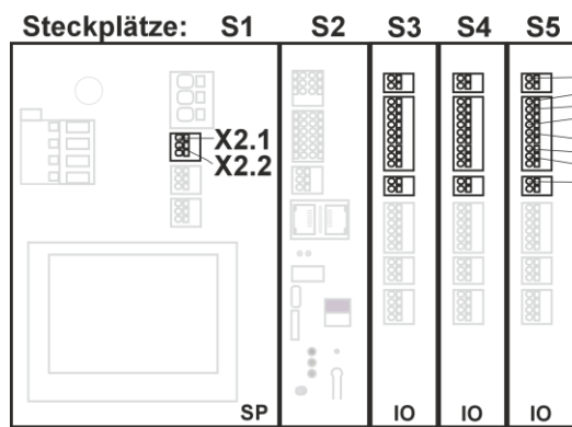
a) RWA-Zentrale mit drei Input/Output-Modulen
