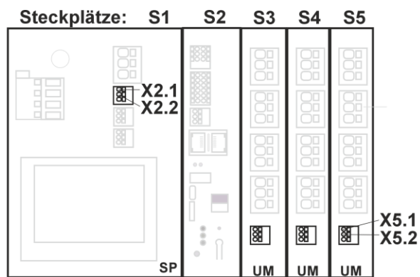
b) RWA-Zentrale mit drei Motormodulen
